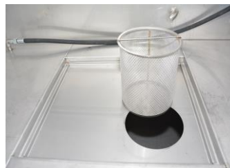
Herausnehmbarer Grobfilter
